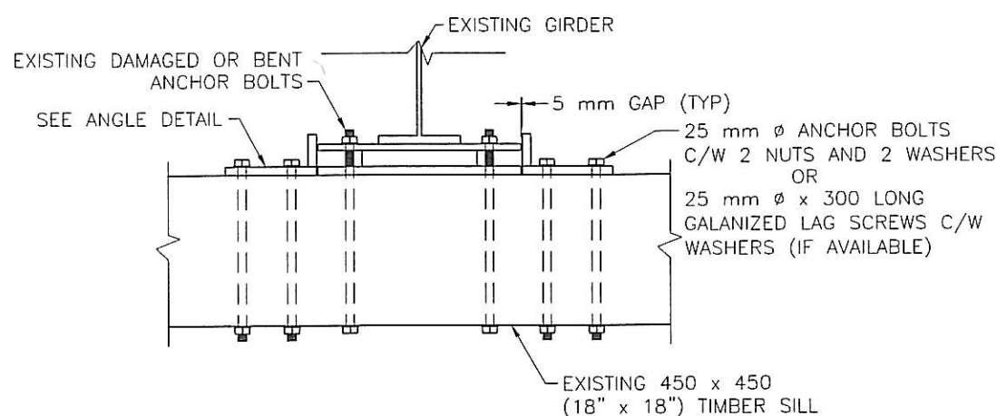
EXISTING 1:20
